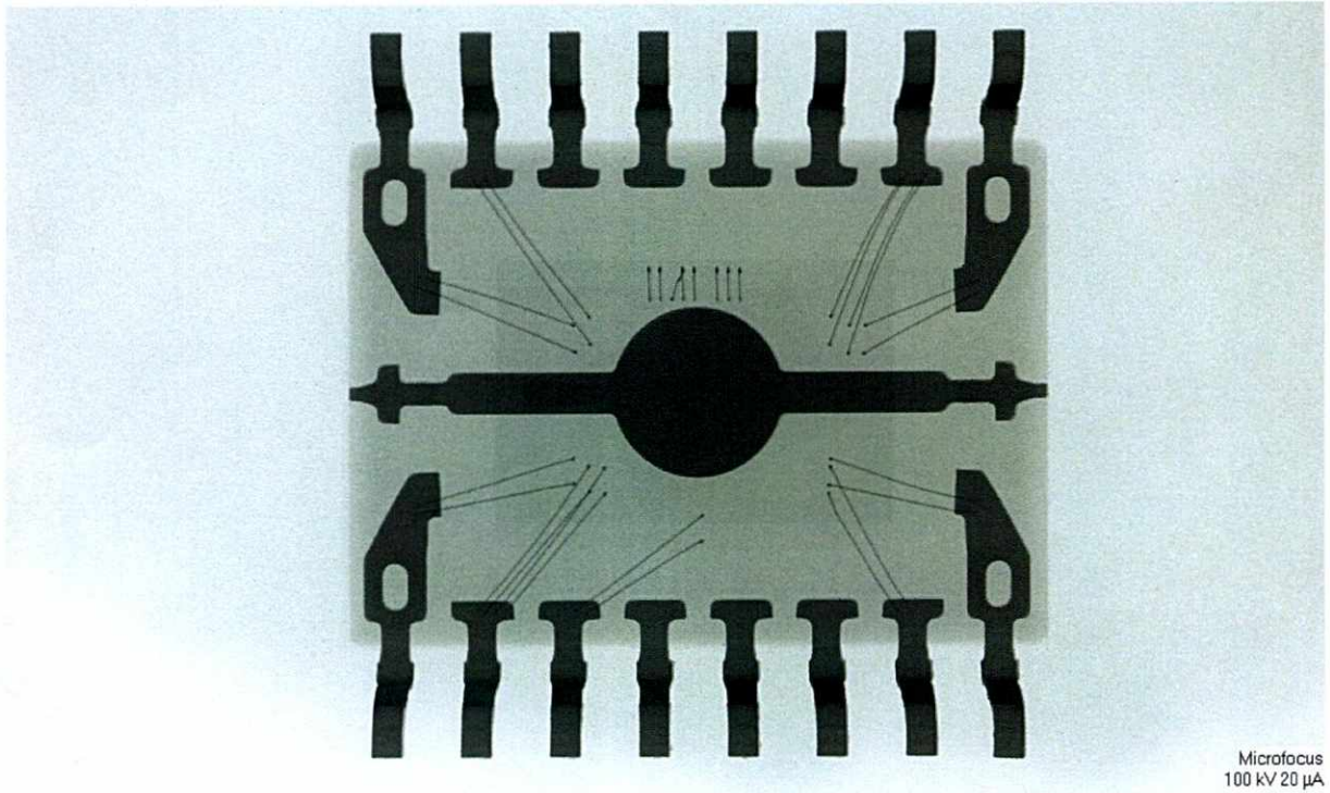
照片编号: X 射线检-1 照片内容: #2 Y 方向
